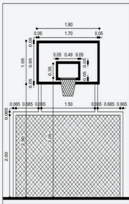
Vista frontal del soporte integrado de baloncesto y microfútbol.
